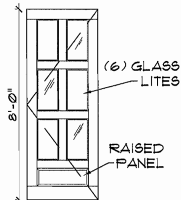
(D) WOOD & GLASS DOOR
